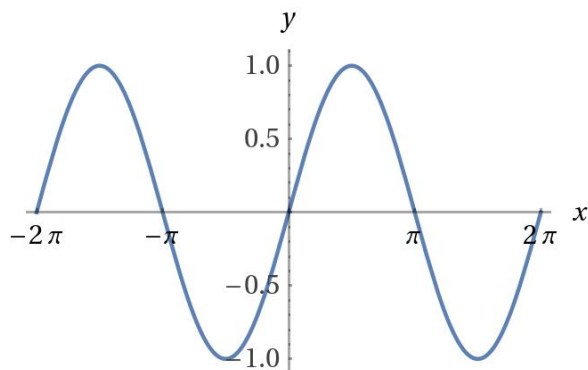
1-сурет. y = \sin(x) функциясының графигі.
