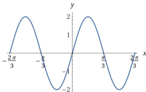
2-сурет. y = 2\sin(3x) функциясының графигі.
